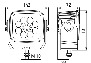
1GA 995 706-521 RokLUME 280N Gen. 2 - ZEROGLARE
