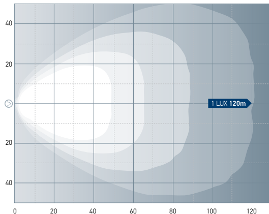
RokLUME 380 - Close Range
