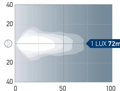
RokLUME 380N - ZEROGLARE
